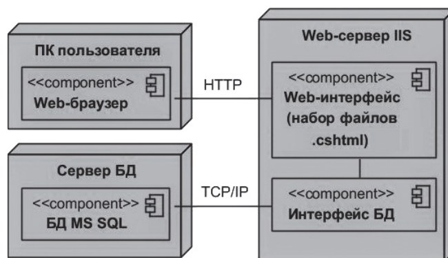
Рис. 7. Диаграмма развертывания
