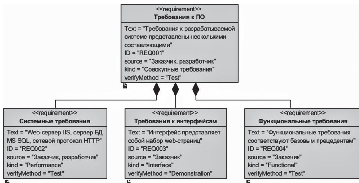
Рис. 1. Диаграмма требований
