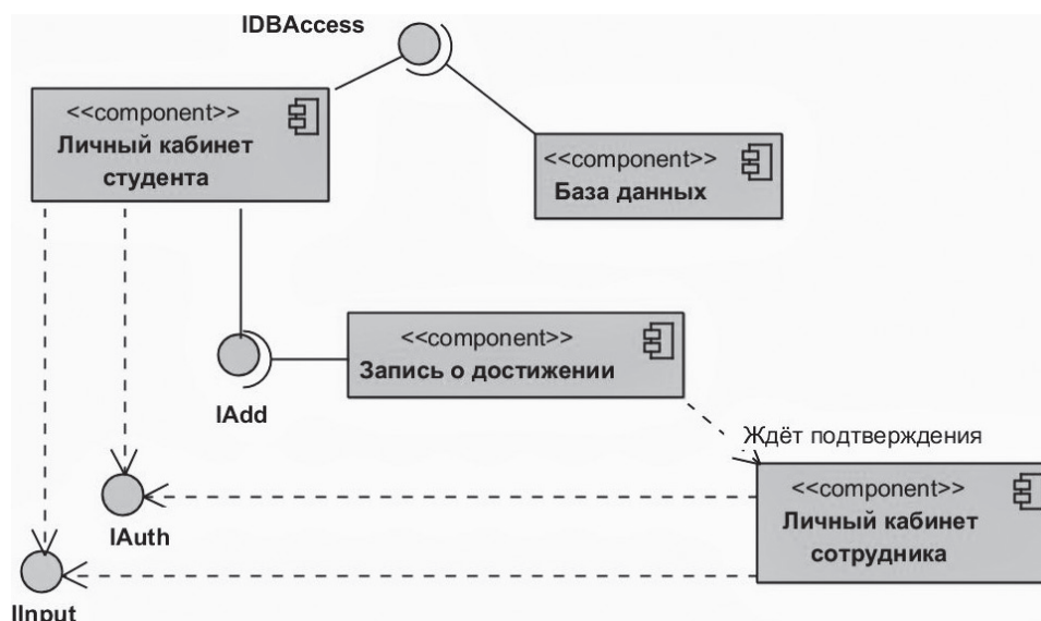
Рис. 6. Диаграмма компонентов
