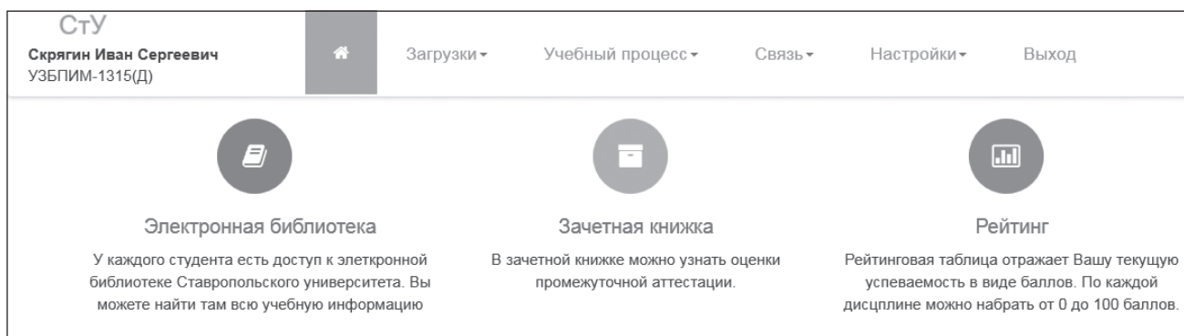
Рис. 4. Интерфейс студента
