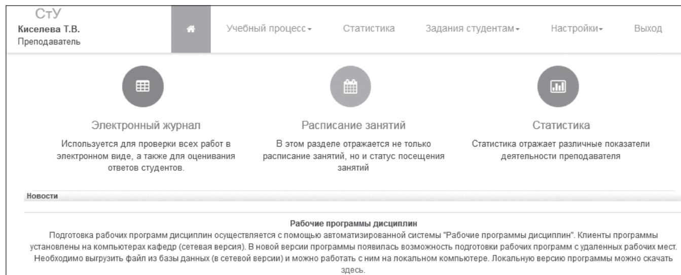
Рис. 5. Интерфейс преподавателя
